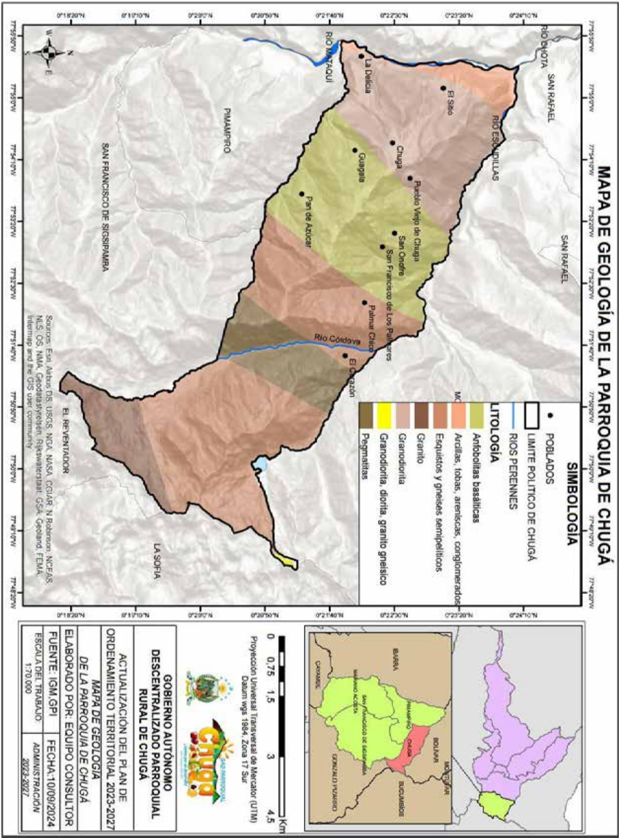
Mapa 5. Geología de Chugá
